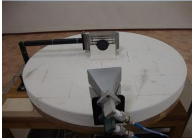
Reflexiós mérőpad radarelnyelés méréséhez
