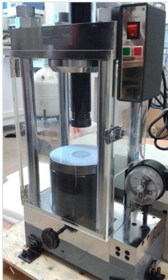
Elektromos-hidraulikus présgép (60 t)
